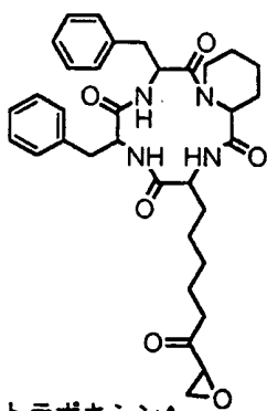
トラボキシシンA
